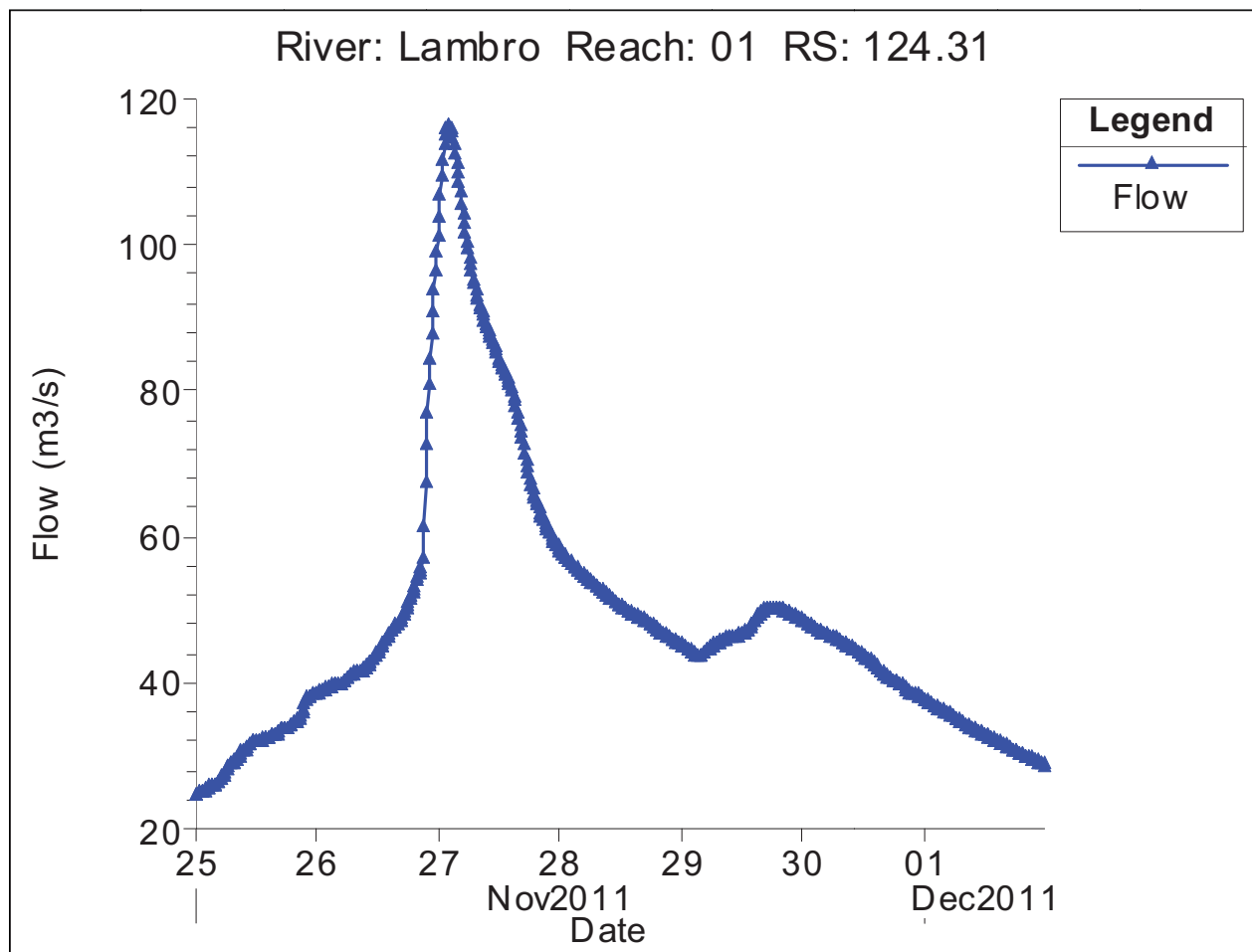
Figura 22 – Idrogramma sezione 124.31 di Hec-Ras ricavato dal modello di MIKE dello studio AdB
