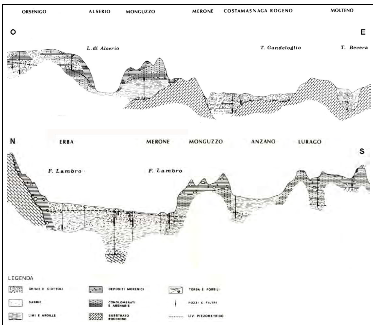
Figura 28: Sezioni idrogeologiche E-O e N-S
