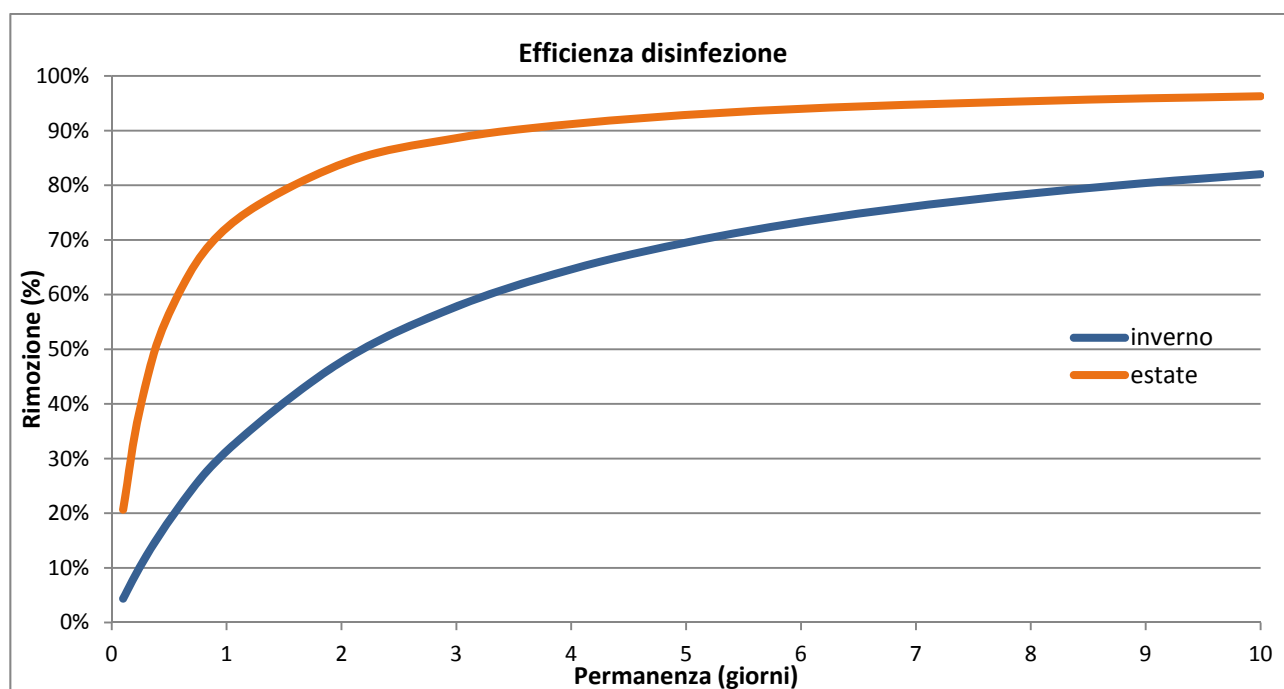
Figura 23 – Rimoziioni percentuali dei batteri (coliformi fecali)
